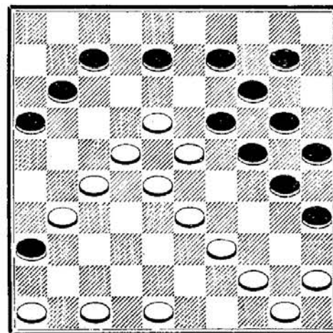
N° 645 — Problème par Voyant Père.
